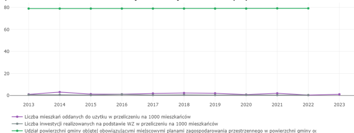
Rysunek 51. Stosowanie instrumentów planowania przestrzeni w Kętrzynie - wskaźniki
