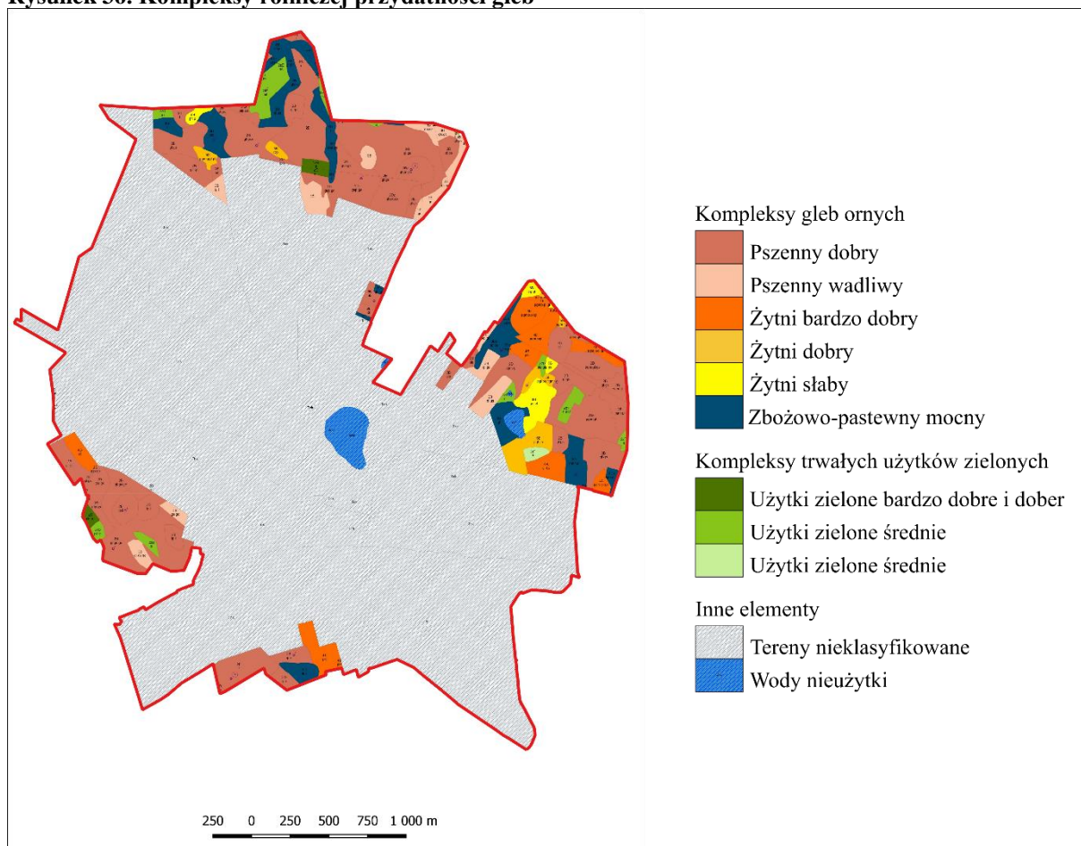
Rysunek 36. Kompleksy rolniczej przydatności gleb
