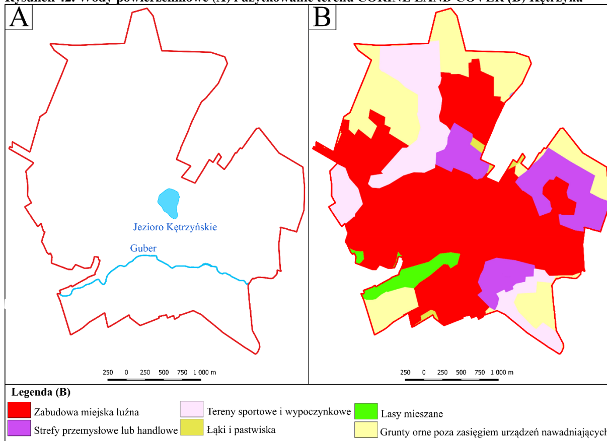
Rysunek 42. Wody powierzchniowe (A) i użytkowanie terenu CORINE LAND COVER (B) Kętrzyna
